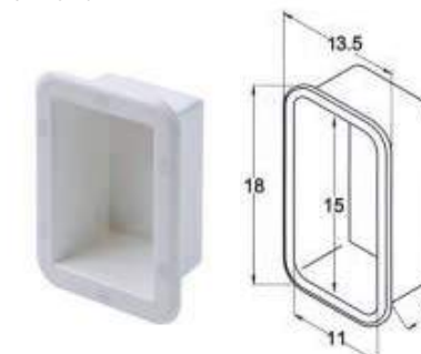
10.361 ΝΤΟΥΛΑΠΙ ΜΙΚΡΟ
