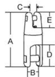
ΣΤΡΙΦΤΑΡΙ
