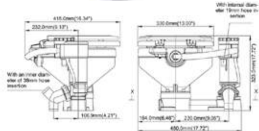
SEAFLO N.T.
