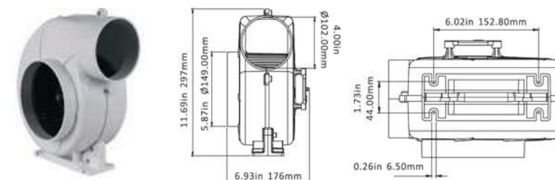
15.188A ΑΕΡΑΓΩΓΟΣ ΒΤ 320FM 12V Ø100mm ΜΕ ΒΑΣΗ 15.188B ΑΕΡΑΓΩΓΟΣ ΒΤ 320FM 24V Ø100mm ΜΕ ΒΑΣΗ
