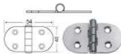
93.132 ΜΕΝΤΕΣΕΣ ΟΒΑΛ
