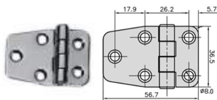
93.122 - ΜΕΝΤΕΣΕΣ 5 ΤΡΥΠΕΣ
