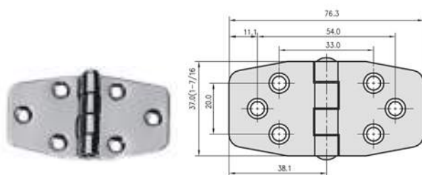
93.123 - ΜΕΝΤΕΣΕΣ 6 ΤΡΥΠΕΣ
