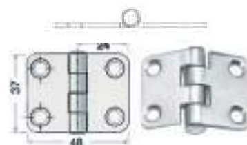
93.146 ΜΕΝΤΕΣΕΣ 4 ΤΡΥΠΕΣ ΠΑΡΑΛΛ/ΜΟΣ
