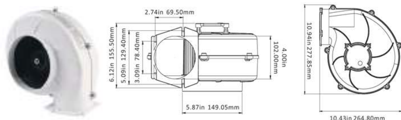
15.187A ΑΕΡΑΓΩΓΟΣ ΒΤ 320FM 12V Φ100mm
