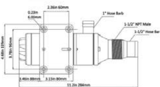
16.530 - ΑΝΤΛΙΑ ΛΥΜΑΤΩΝ MACERATOR 12V 16.550 - ΑΝΤΛΙΑ ΛΥΜΑΤΩΝ MACERATOR 24V
