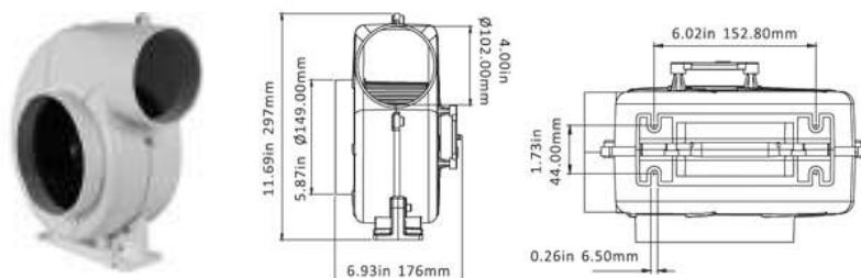
15.188A ΑΕΡΑΓΩΓΟΣ ΒΤ 320FM 12V Φ100mm ΜΕ ΒΑΣΗ
