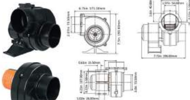
15.193 - ΑΕΡΑΓΩΓΟΣ ΣΑΛΙΓΚΑΡΙ 130 CMF Φ76mm 12V
