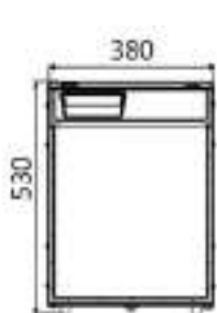
91.071 ΨΥΓΕΙΟ FRIGO 50lit 12-24V
