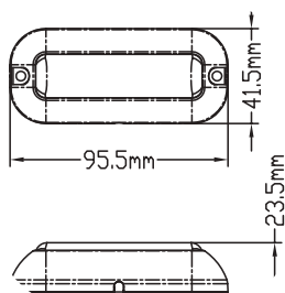
ΦΩΣ ΥΠΟΒΡΥΧΙΟ ΣΤΕΝΟ INOX LED 10-30V 95x40mm 100LM 14.270 ΜΠΛΕ 14.271 ΛΕΥΚΟ
