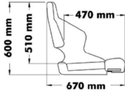
93.100 ΚΑΘΙΣΜΑ ΜΕ FLIP UP Η52 ΜΗΧΑΝΙΣΜΟ
