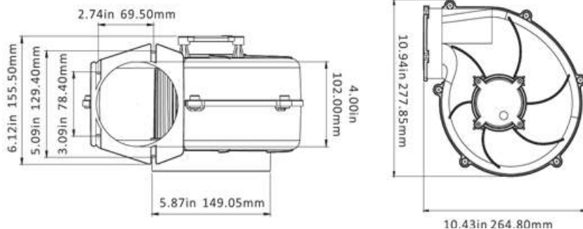
15.187A ΑΕΡΑΓΩΓΟΣ ΒΤ 320FM 12V Φ100mm 15.187B ΑΕΡΑΓΩΓΟΣ ΒΤ 320FM 24V Φ100mm
