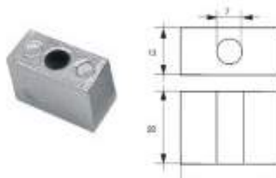
50.257 ΑΝΟΔΙΟ TOHATSU 40÷140HP MEGA3C7-60218-1
