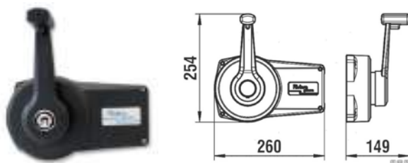
81.309 ΧΕΙΡΙΣΤΗΡΙΟ ΠΛΑΙΝΟ ΜΗΧΑΝΗΣ
