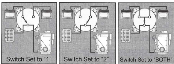
90.034 ΔΙΑΚΟΠΤΗΣ ΜΠΑΤΑΡΙΑΣ ΜΚ2 B0TH ΓΙΑ 2 ΜΠΑΤΑΡΙΕΣ ΣΥΝΕΧΟΜΕΝΟ 300A/max 450A
