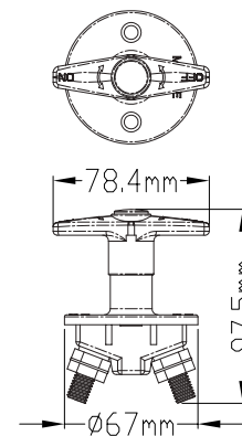
14.127 ΔΙΑΚΟΠΤΗΣ ΜΠΑΤΑΡΙΑΣ 1000A/ON-OFF 1000A
