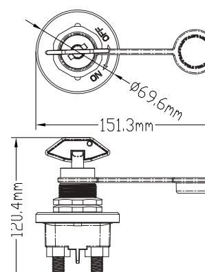
14.129 ΔΙΑΚΟΠΤΗΣ ΜΠΑΤΑΡΙΑΣ ON-OFF B.T. 250A/ ΜΕ ΚΛΕΙΔΙ INOX max 2000A
