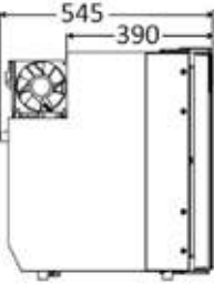
91.072 ΨΥΓΕΙΟ FRIGO 85lit 12-24V
