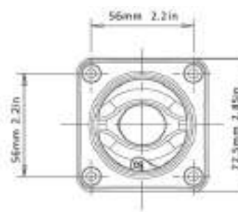
14.129 ΔΙΑΚΟΠΤΗΣ ΜΠΑΤΑΡΙΑΣ ON-OFF B.T. 250A/ ΜΕ ΚΛΕΙΔΙ INOX max 2000A
