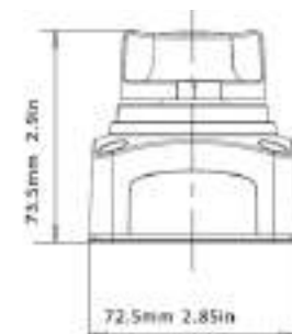
14.129 ΔΙΑΚΟΠΤΗΣ ΜΠΑΤΑΡΙΑΣ ON-OFF B.T. 250A/ ΜΕ ΚΛΕΙΔΙ INOX max 2000A
