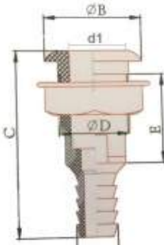
10.341 ΑΝΕΠΙΣΤΡΟΦΗ ΒΑΛΒΙΔΑ Ø40mm
