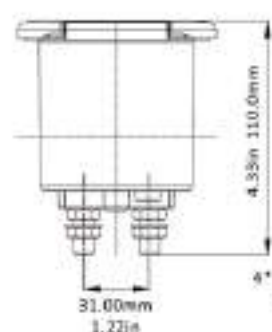
14.126 ΔΙΑΚΟΠΤΗΣ ΜΠΑΤΑΡΙΑΣ ΜΕ ΚΛΕΙΔΙ ΧΩΝΕΥΤΟΣ 100A/max1000A
