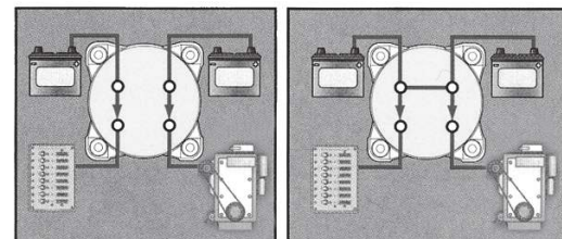
90.035 ΔΙΑΚΟΠΤΗΣ ΜΠΑΤΑΡΙΑΣ ΜΚ3 B0TH ΓΙΑ 2 ΜΠΑΤΑΡΙΕΣ 300A/450A
