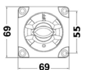
14.123 ΔΙΑΚΟΠΤΗΣ ΓΙΑ 2 ΜΠΑΤΑΡΙΕΣ B0TH ΜΙΚΡΟΣ 100A max 300A
